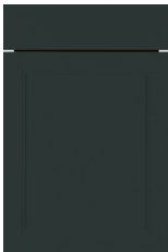
graphite (A 881)
